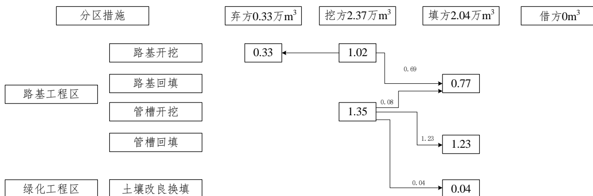
图 2-7 土石方平衡流向框图
