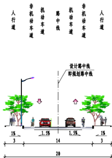
图 2-3 道路横断面图
